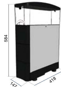
UNITE RESERVOIR D'EAU UNIDAD TANQUE DE AGUA
